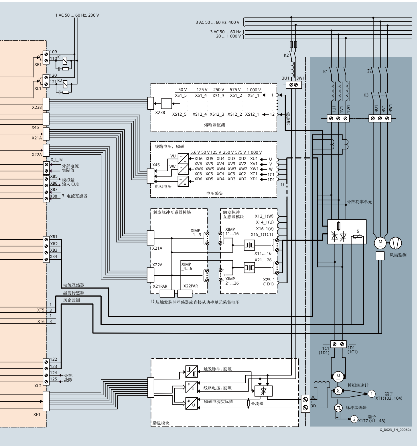
电路图 (续)
