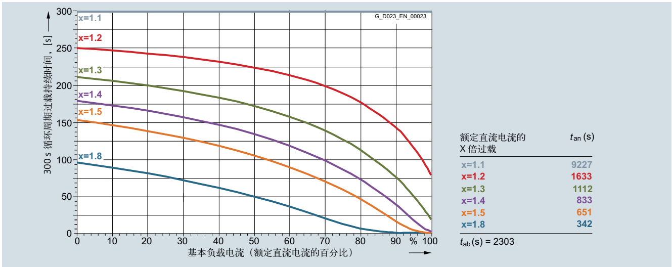
6RA8013-6DV62-0AA0 15 A/ 四象限运行, 400V; 6RA8013-6FV62-0AA0 15A/ 四象限运行, 480V
