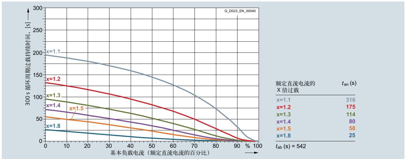
6RA8087-6DS22-0AA0 850 A/ 两象限运行, 400 V,
