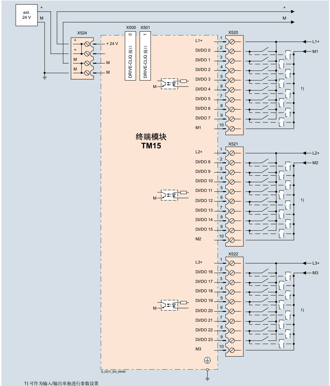
TM15 终端模块连接示例
