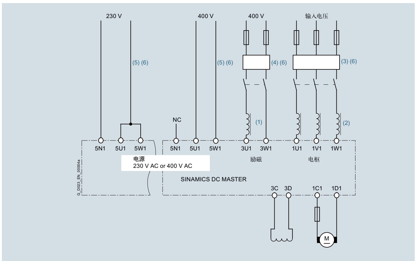
电抗器和无线电干扰滤波器的布置
