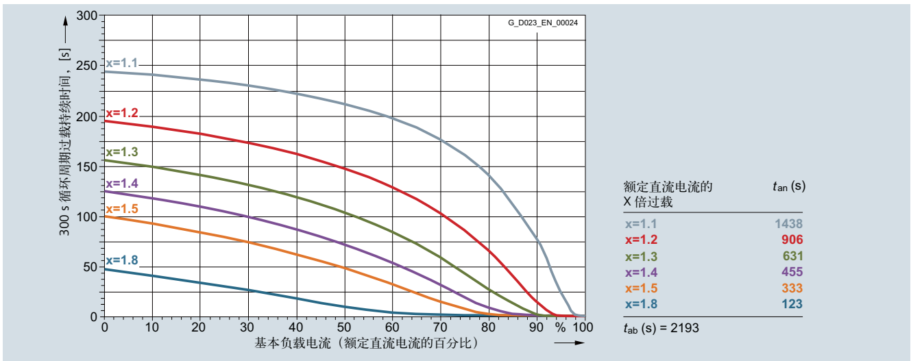
6RA8018-6DV62-0AA0 30 A/ 四象限运行, 400V; 6RA8018-6FV62-0AA0 30 A/ 四象限运行, 480V
