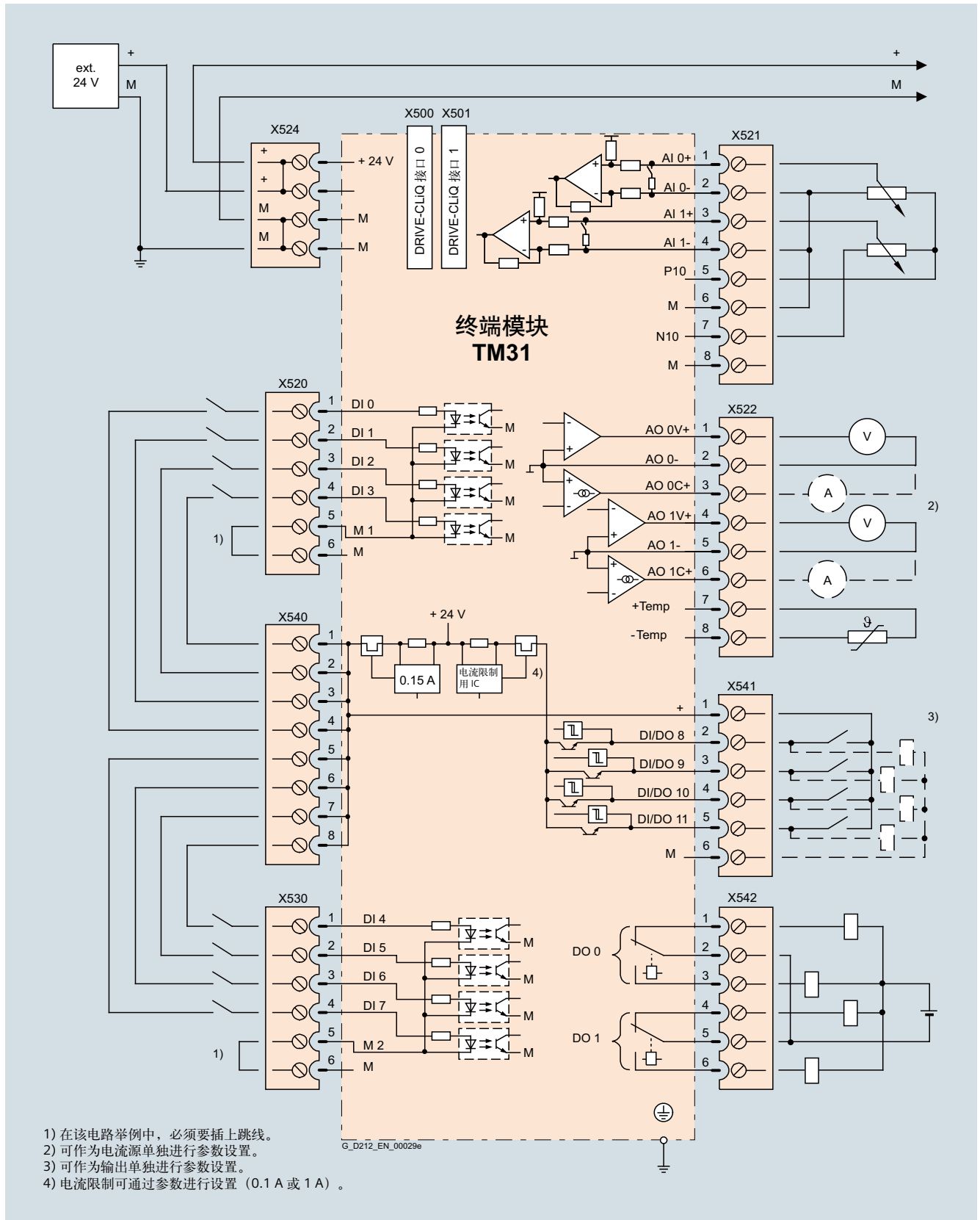
TM31 终端模块连接示例
