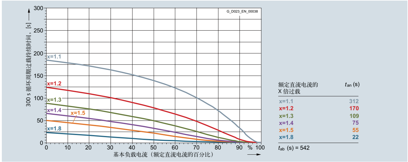
6RA8086-6KS22-0AA0 720 A/ 两象限运行, 690 V
